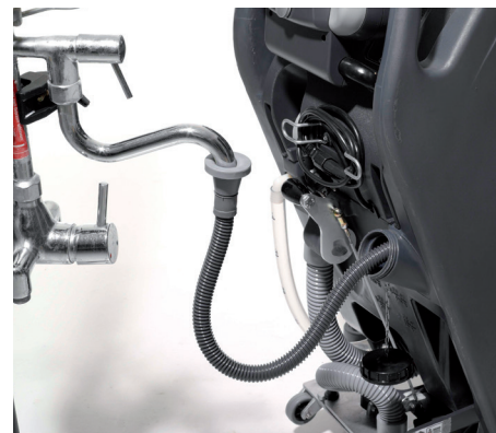
Sistema di riempimento facilitato del serbatoio soluzione con tubo allungabile (opzionale) che consente di riempire il serbatoio anche dalla parte posteriore della macchina
